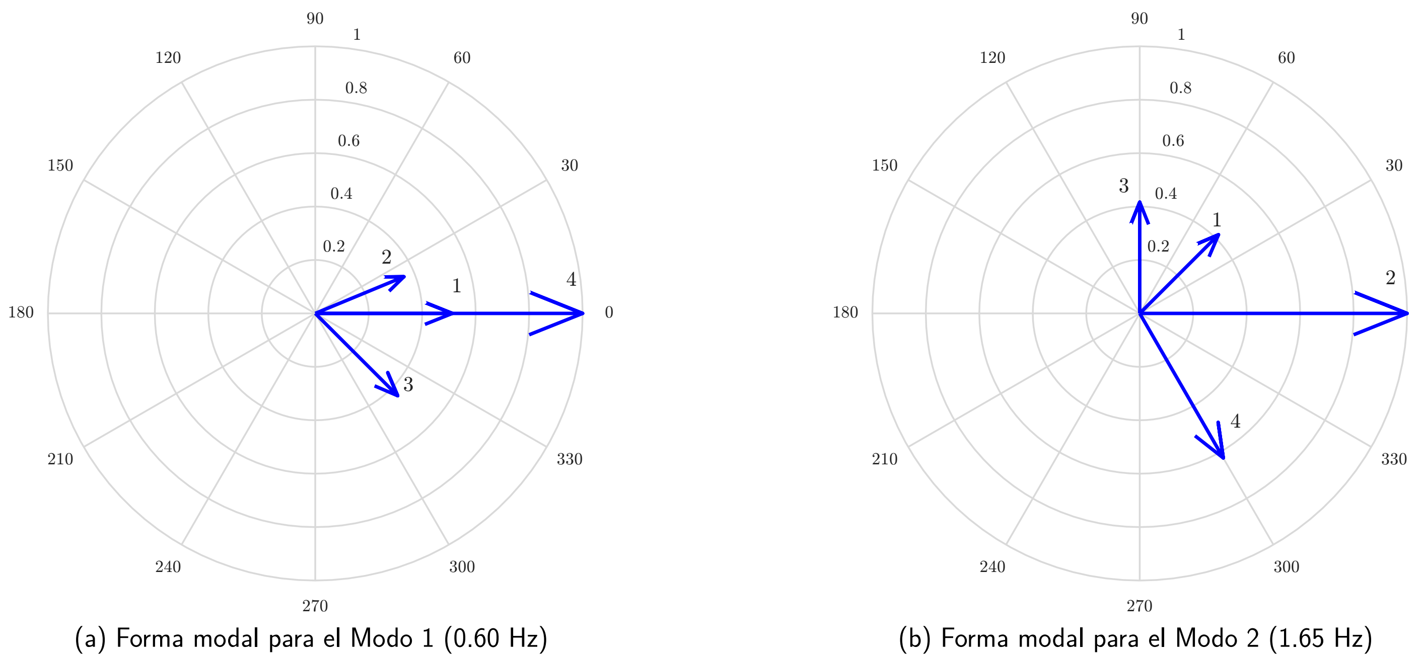
(a) Forma modal para el Modo 1 (0.60 Hz)
