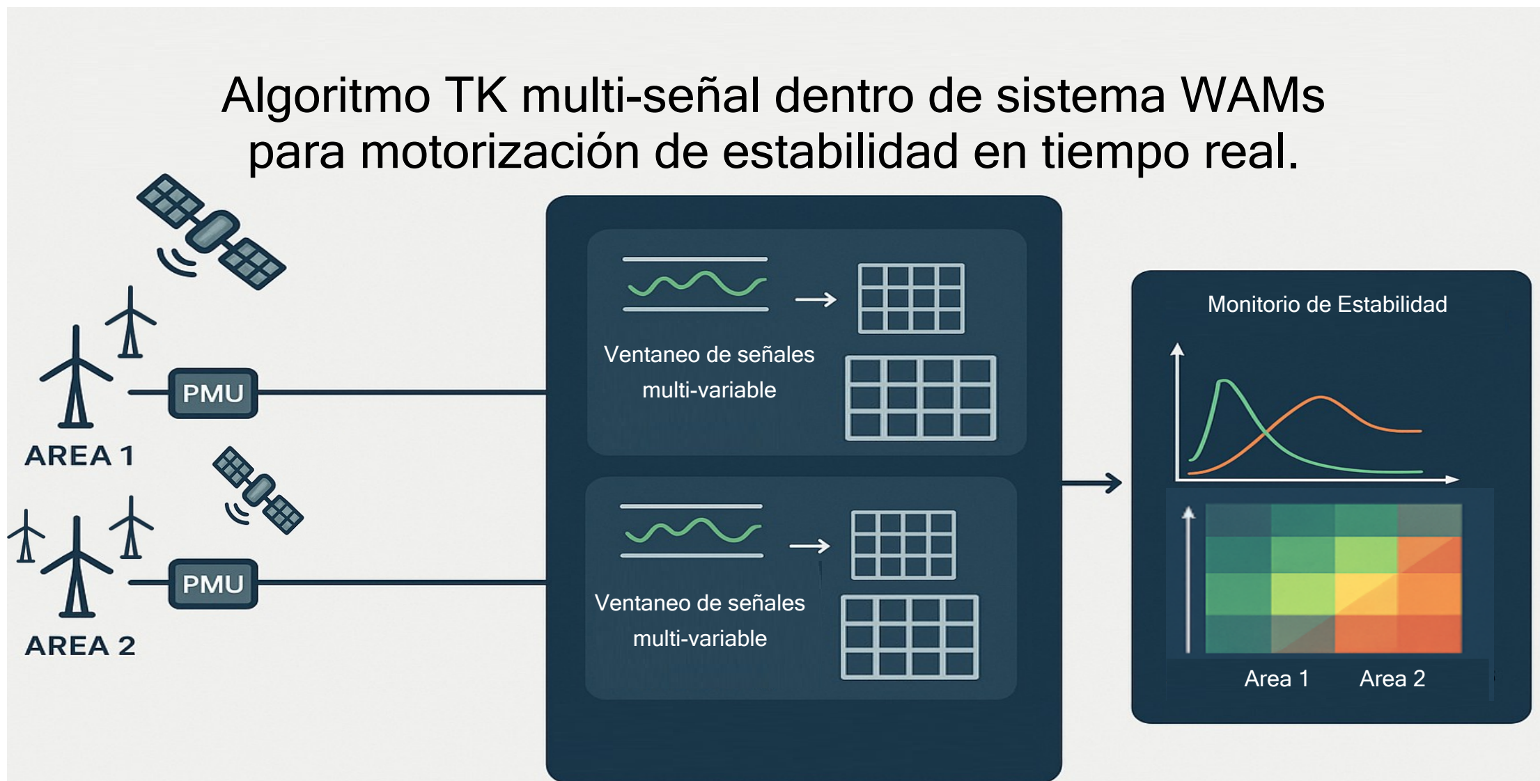
Figura 1: Diagrama de flujo del algoritmo Multi-TK propuesto.
