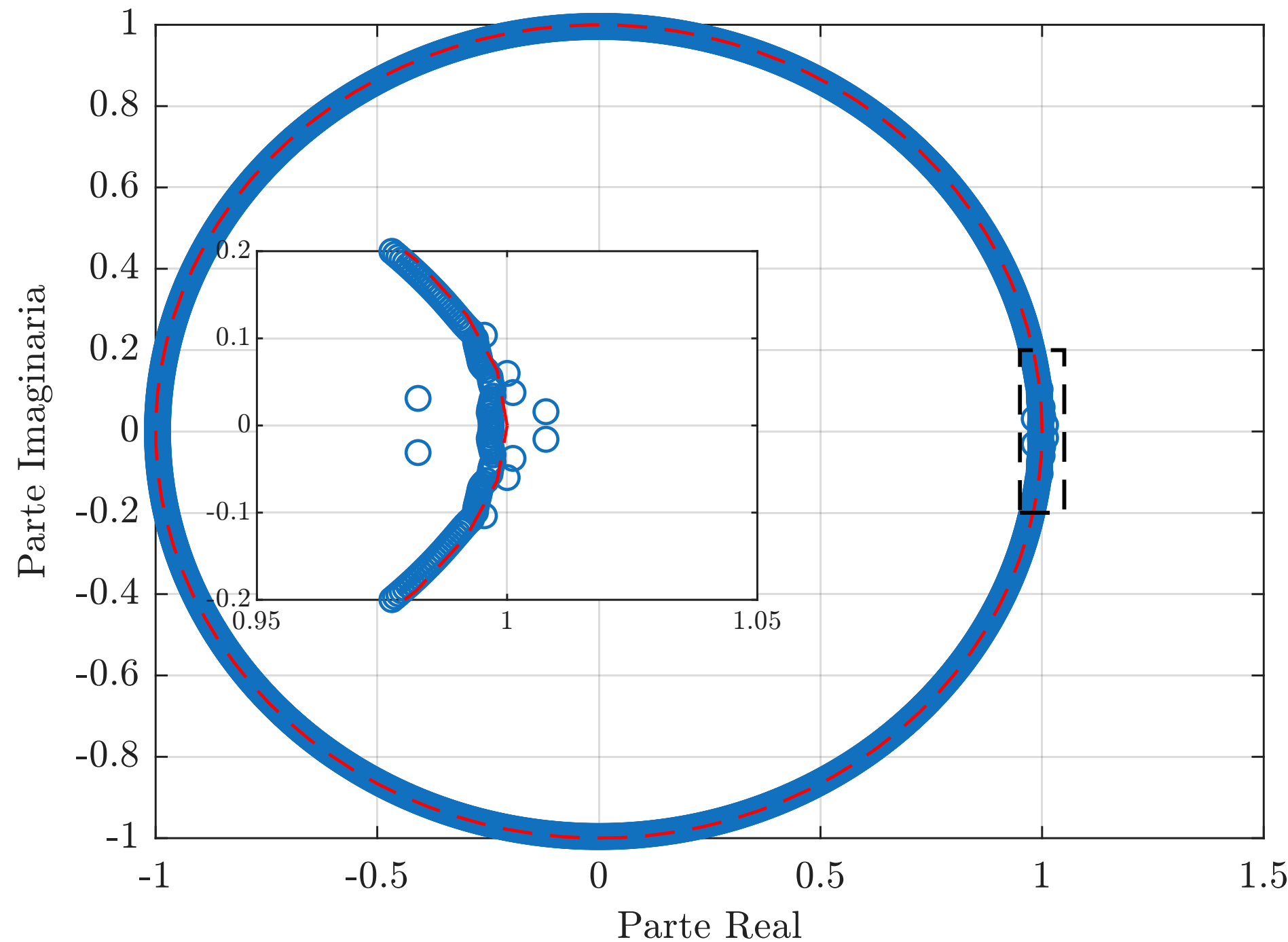
Figura 2: Identificación de polos en el plano Z.
