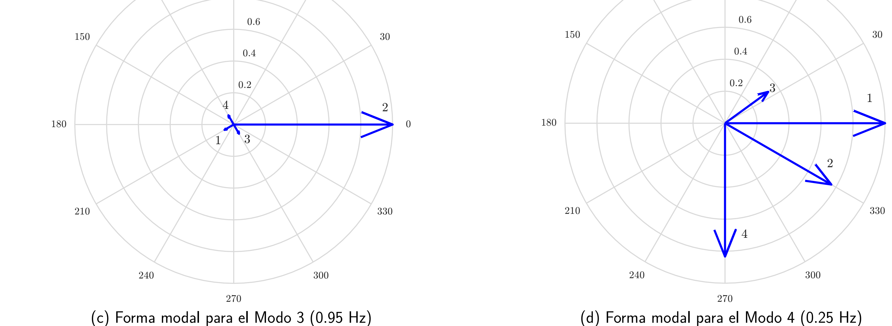
Figura 4: Formas modales estimadas por el algoritmo TK
